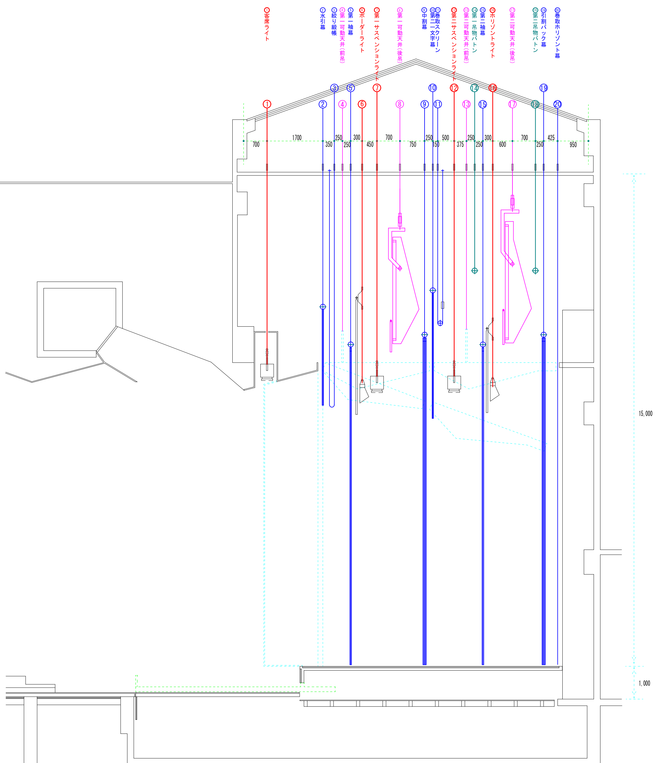
多目的ホール断面図 A3 1/70
